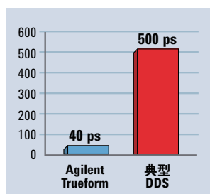
抖动
